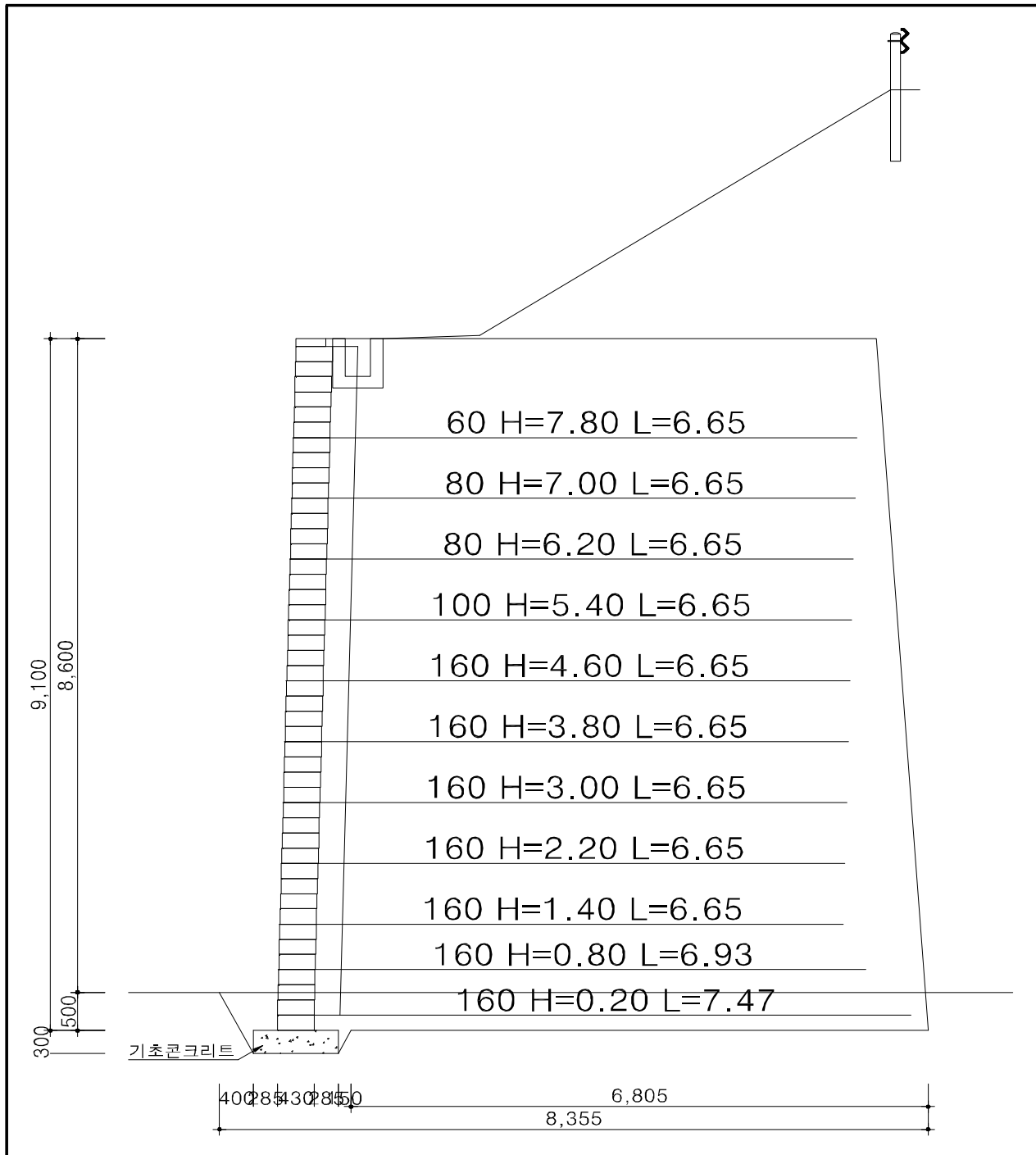
【그림 69.9】 검토단면도
